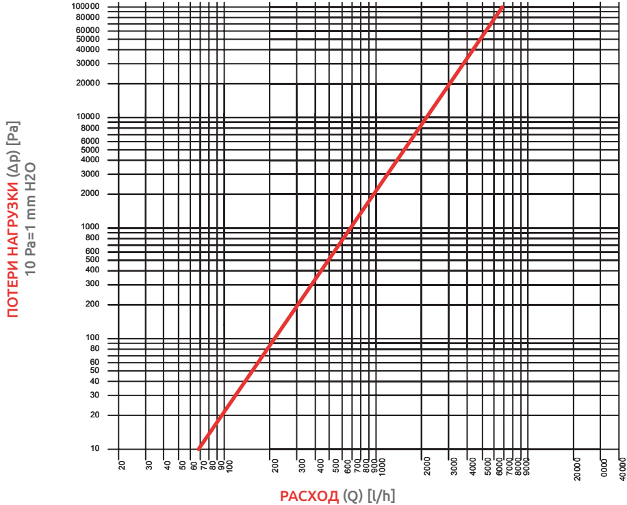
НАСОСНЫЕ ГРУППЫ Арт. R003 ДИАГРАММА ПОТЕРИ НАГРУЗКИ
