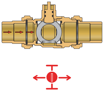
СЕРВОМОТОР ЗАКРЫТ
