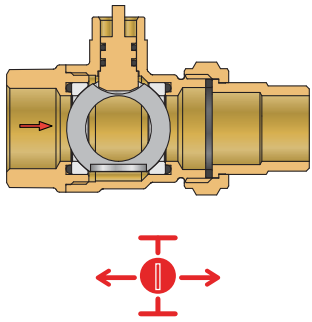
СЕРВОМОТОР ЗАКРЫТ
