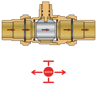
СЕРВОМОТОР ОТКРЫТ
