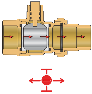
СЕРВОМОТОР ОТКРЫТ
