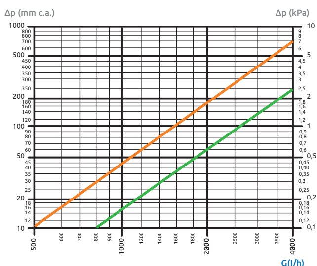
GRAFICO COLLETTORE
