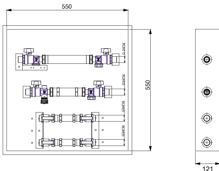
Dima chiusa
