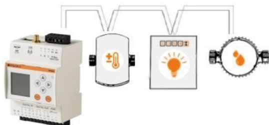
Topologia di linea
